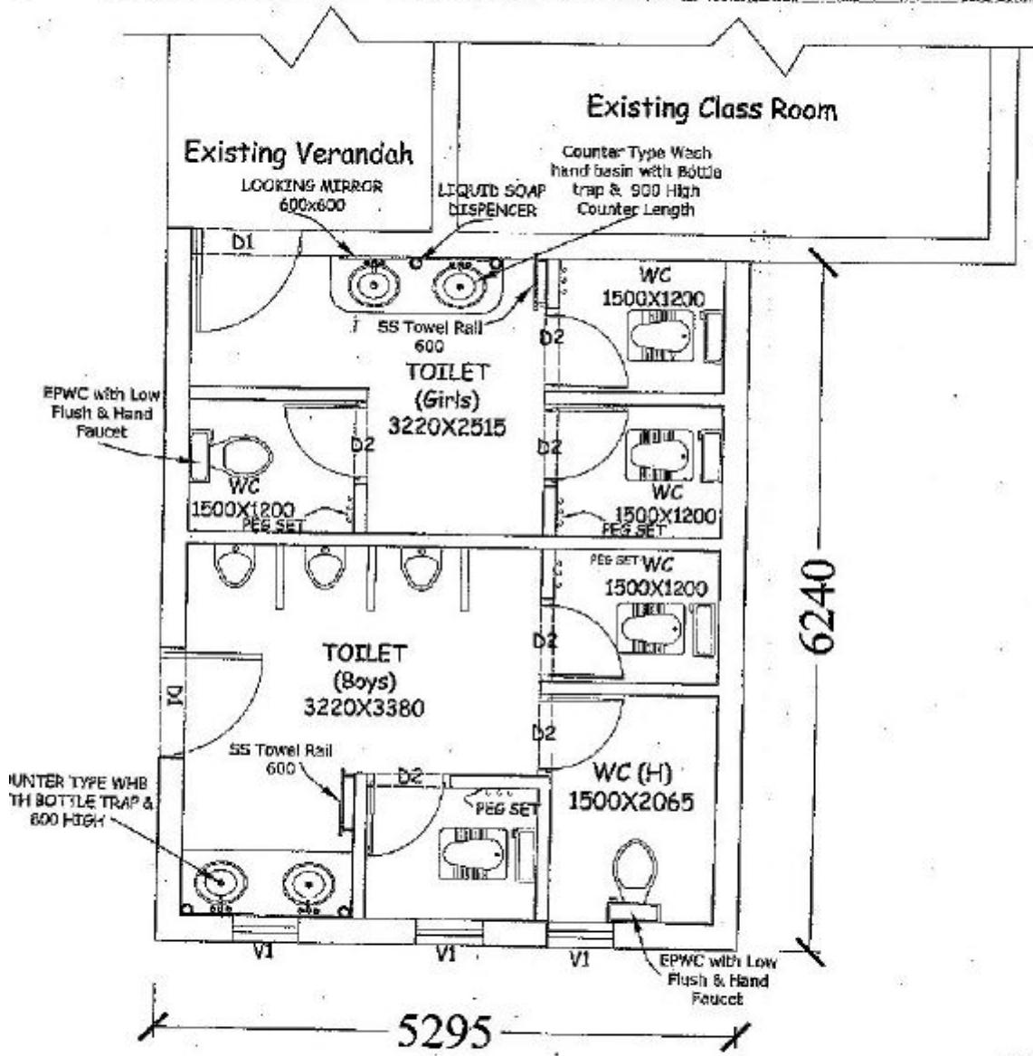
DW-01 PLAN
